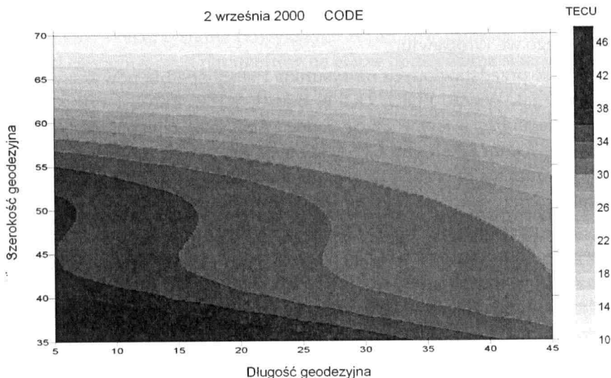
Rys. 3. Model stanu jonosfery GIM opracowany w centrum analiz CODE dla obszaru Europy z godz. 12:00 z dnia 2 września 2000 roku
